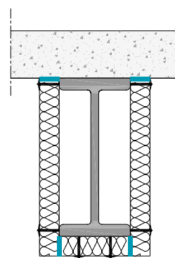
Punti di applicazione della colla CONLIT
