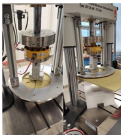
Immagini prove di estrazione
