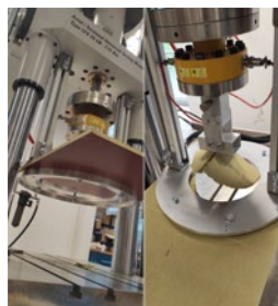
Immagini prove di estrazione
