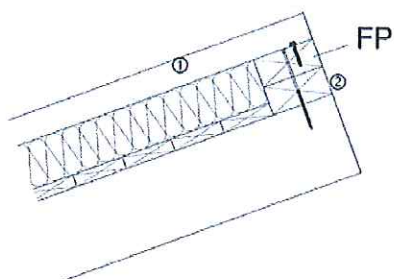
Unterkonstruktion: Holz Festpunkt (FP): Holzbauteil
