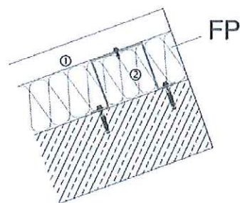
Unterkonstruktion: Beton oder Porenbeton Festpunkt (FP): Kanteil aus Stahl o.a.
