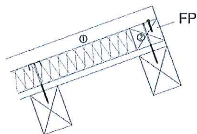
Unterkonstruktion: Holz Festpunkt (FP): Holzbauteil
