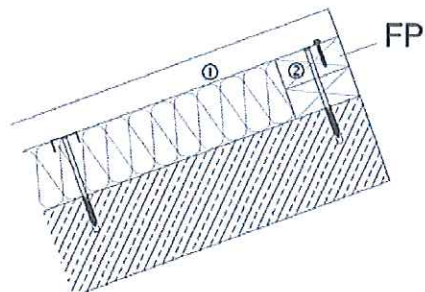
Unterkonstruktion: Beton oder Porenbeton Festpunkt (FP): Holzbauteil
